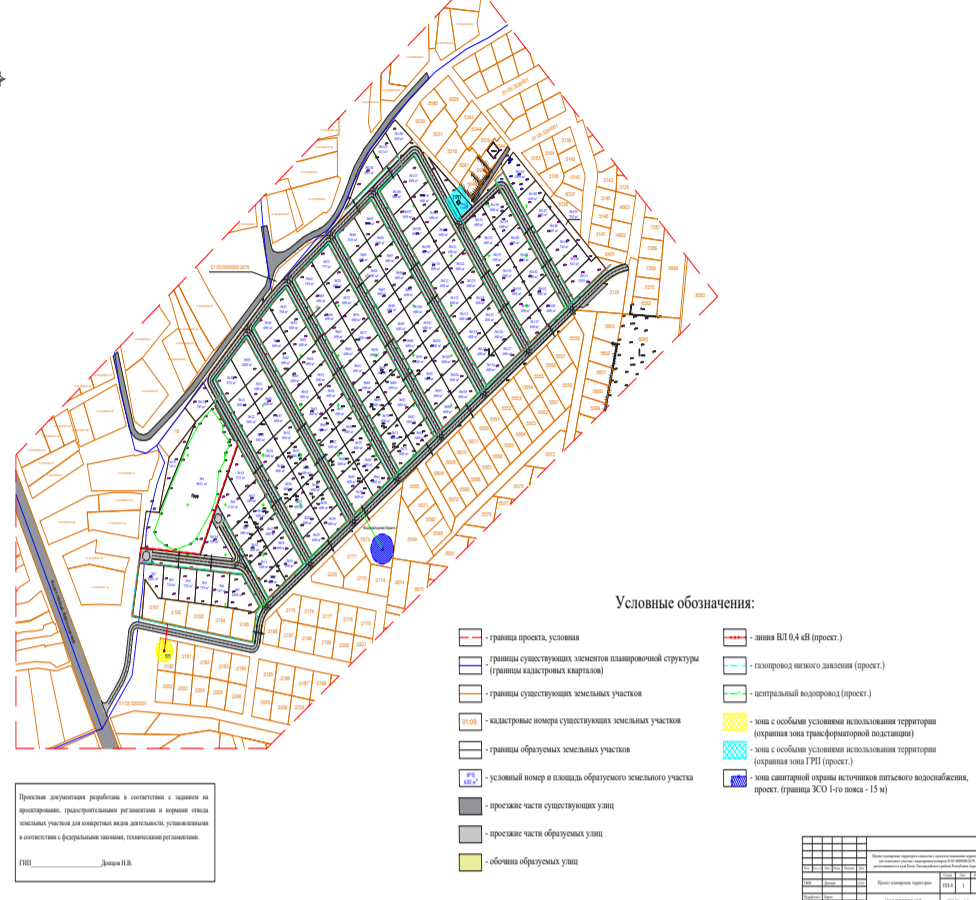
СХЕМА ВЕРТИКАЛЬНОЙ ПЛАНИРОВКИ М 1:1000
